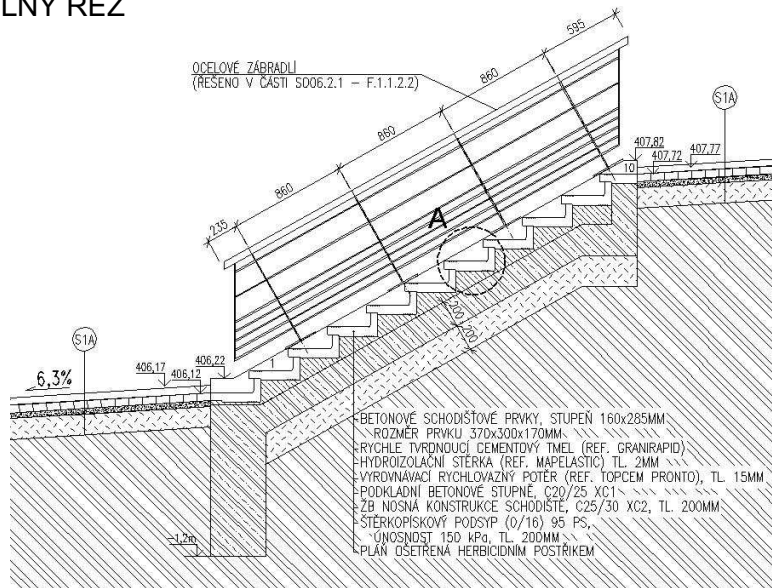
PODÉLNÝ ŘEZ
