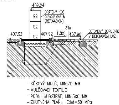
ŘEZ PŘÍČNÝ
