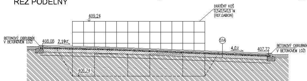
ŘEZ PODÉLNÝ
